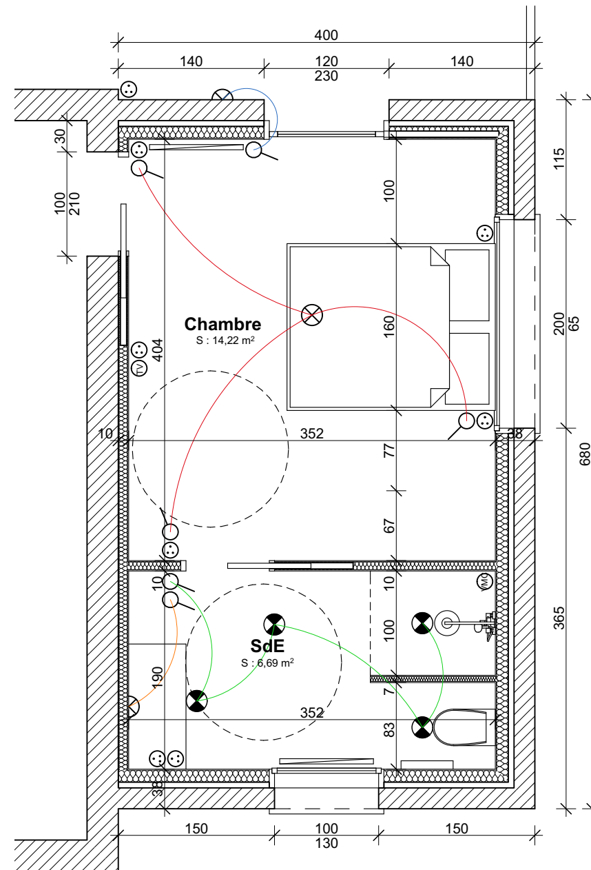
IMPLANTATION - Etat Projet Ech 1/50 - 17/09/2025
