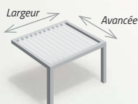
Pergola un module, lames perpendiculaires à la façade Avancée jusqu'à 4000 mm Largeur jusqu'à 5910 mm
